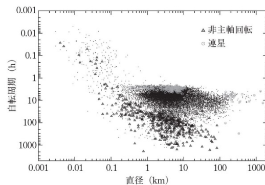
天第3図 小惑星の自転周期 2)
