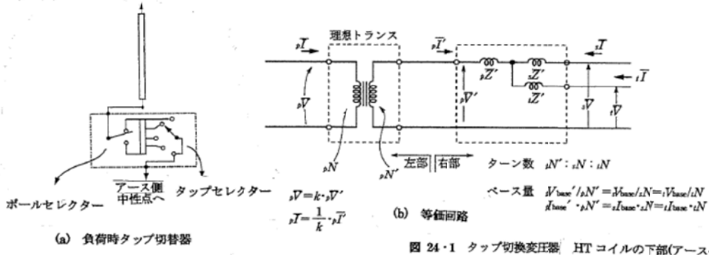
図 24・1 タップ切換変圧器 (HT コイルの下部(アース側)に配置する)
