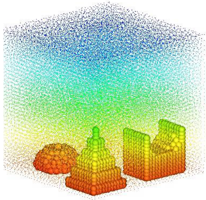
(b) 水および境界粒子の圧力分布
