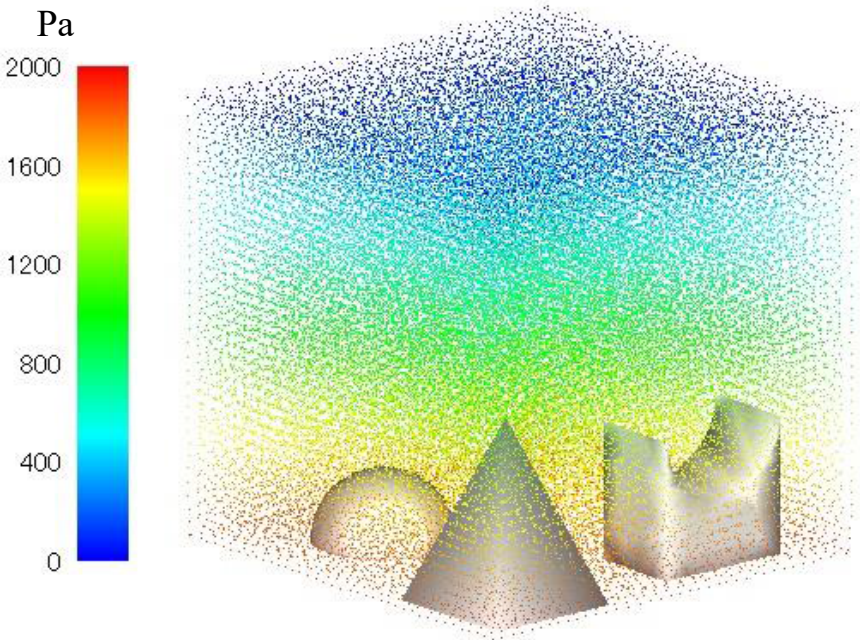
(a) 水粒子の圧力分布
